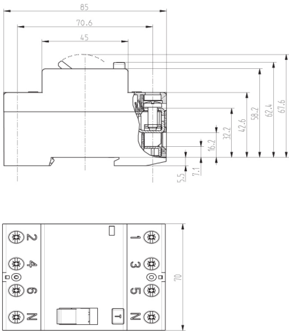
ETI-4 100 A
